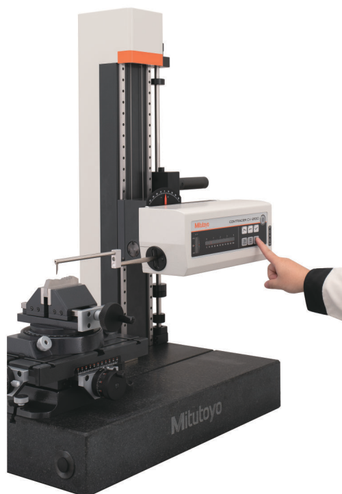
Pohled na CV-2100M4 a přední ovládací panel
